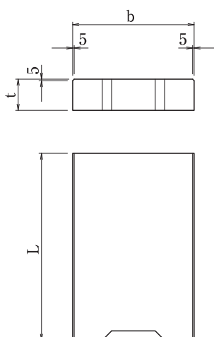
愛知県規格蓋(K種)
